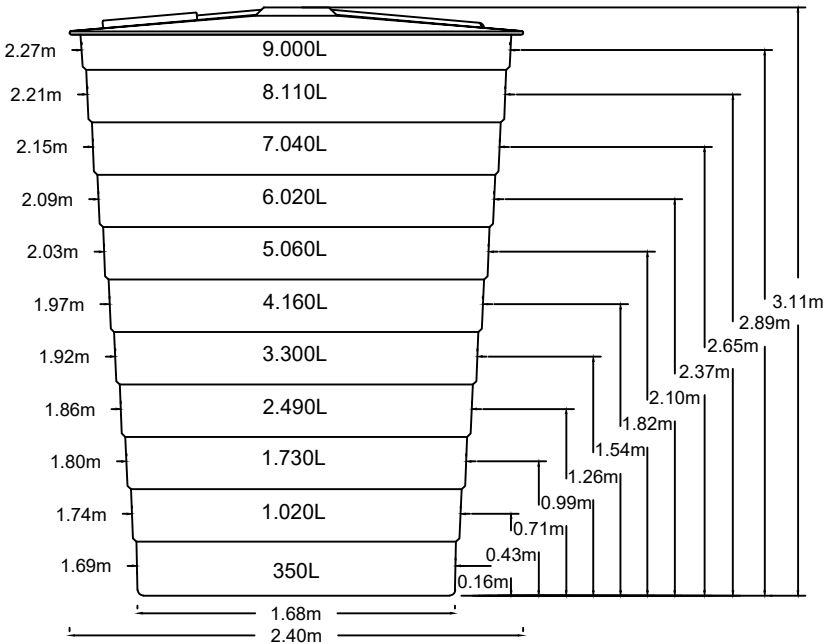
CAIXA PRFV 9000 L
