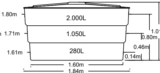
CAIXA PRFV 2000 L
