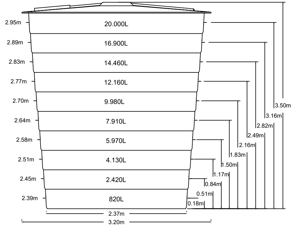
CAIXA PRFV 20000 L
