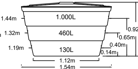
CAIXA PRFV 1000 L
