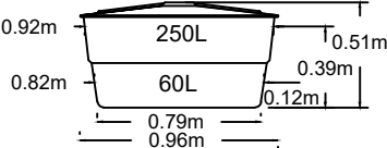
CAIXA PRFV 250 L
