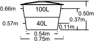
CAIXA PRFV 100 L
