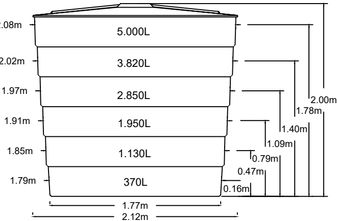
CAIXA PRFV 5000 L
