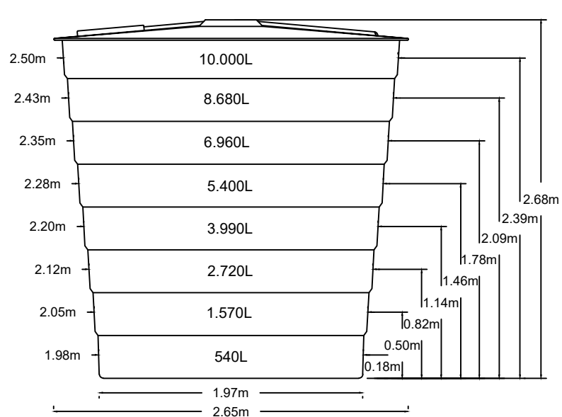
CAIXA PRFV 10000 L
