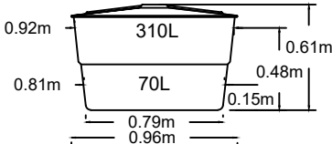
CAIXA PRFV 310 L
