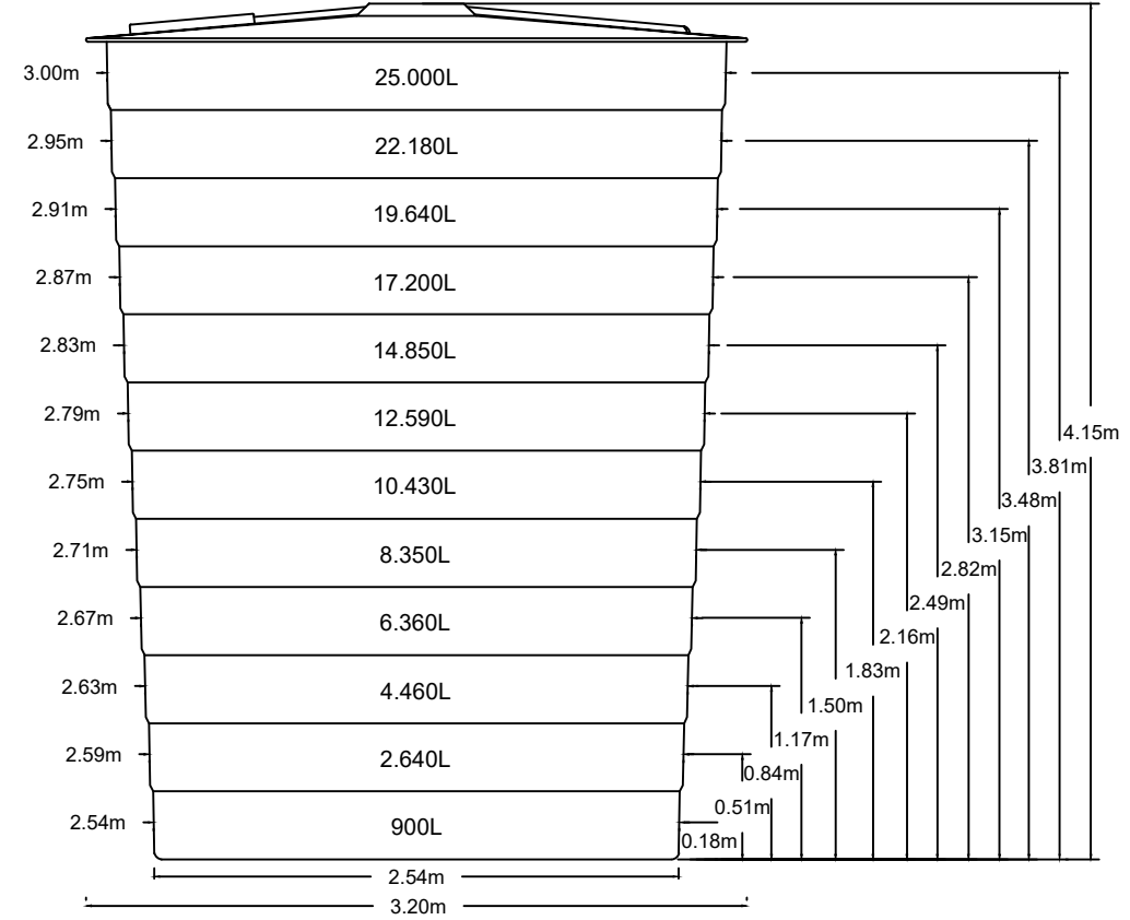
CAIXA PRFV 25000 L
