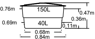
CAIXA PRFV 150 L
