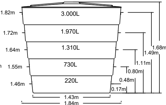
CAIXA PRFV 3000 L
