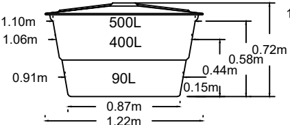
CAIXA PRFV 500 L
