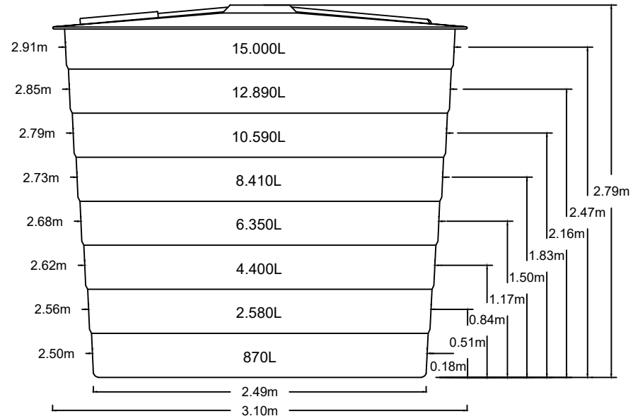
CAIXA PRFV 15000 L
